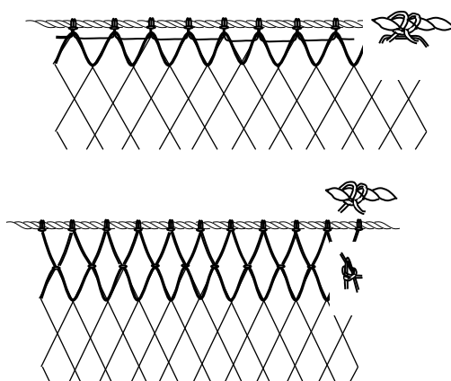
Figura 2.17 Encabalgado en redes con malla grande (Andreev, 1962)
