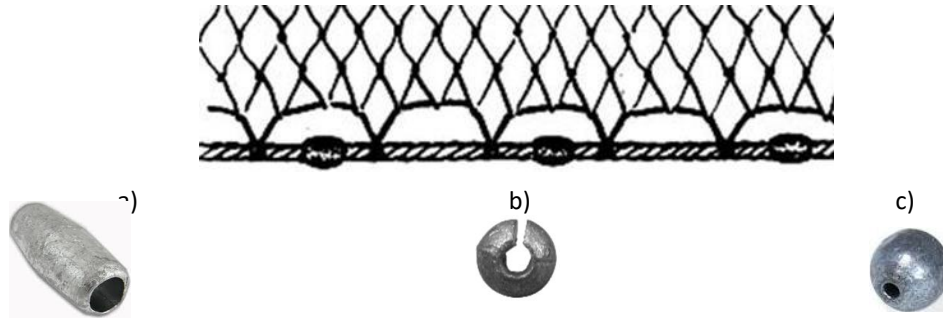
Figura 2.19 Plomos s utilizados en las redes de enmalle; a) Barrilito cerrado, b) Bola abierto c) Esfera cerrado.
