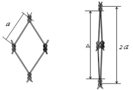
Figura.2.13 Dimensiones principales de una malla
