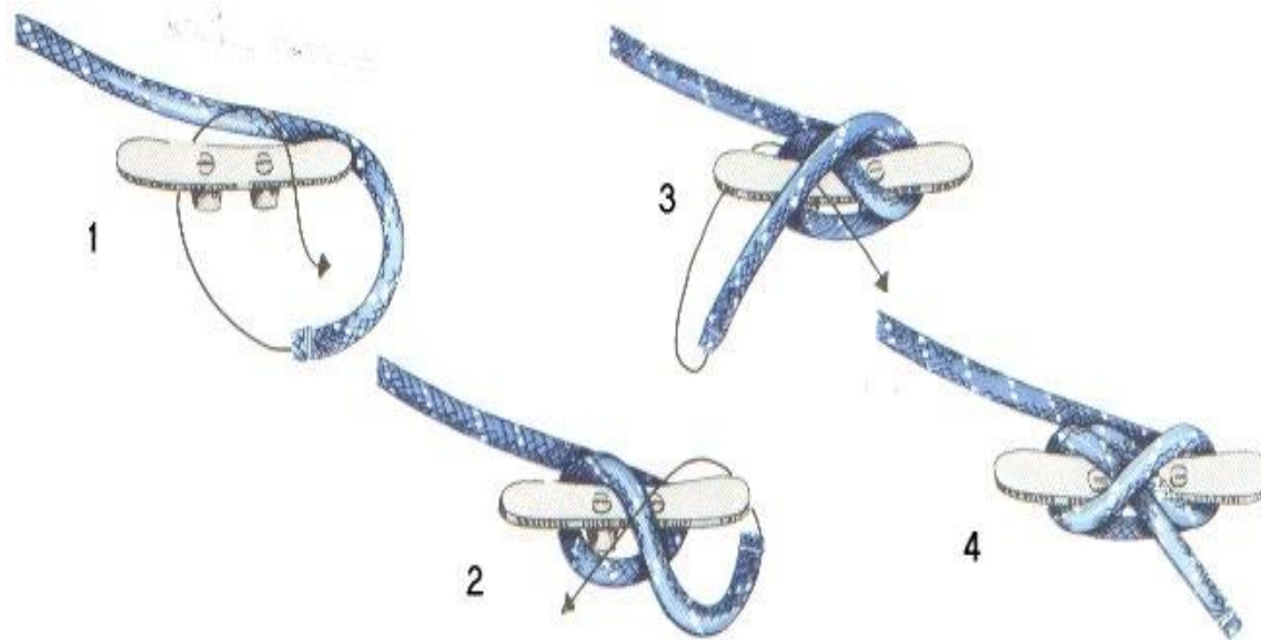
Figura Vuelta de cornamuza
